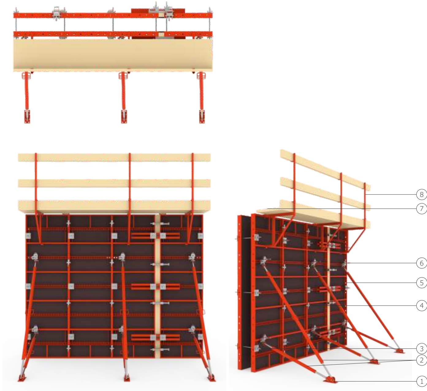
Rapid perde kalıp tipik planı, görünüşü ve kesiti / Rapid wall formwork typical plan, view and section.
