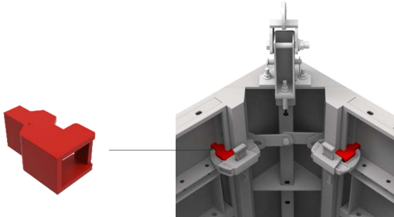
Rapid - Rapido Bağlantı Elemanı Rapid - Rapido Connector
