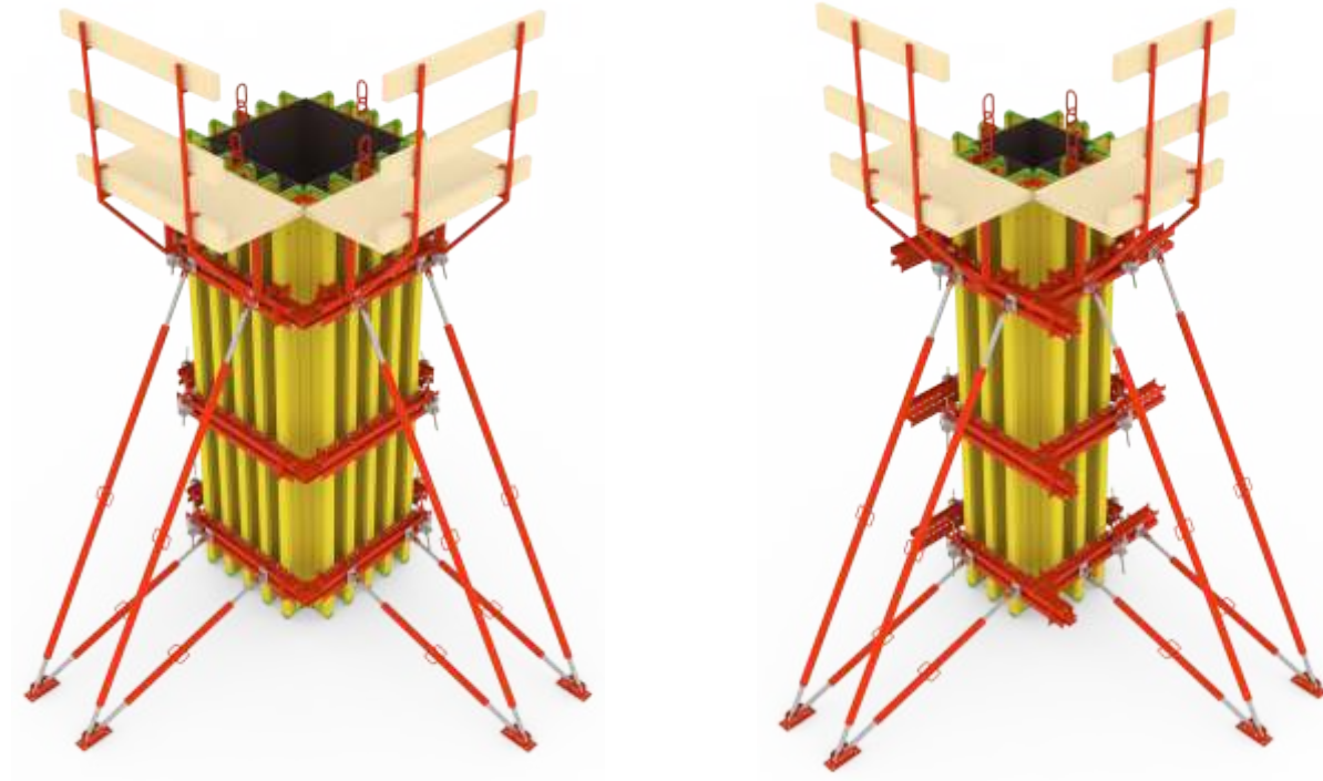
Aynı kuşaklarla yapılan farklı ebatlardaki kolon kalıbı örnekleri
